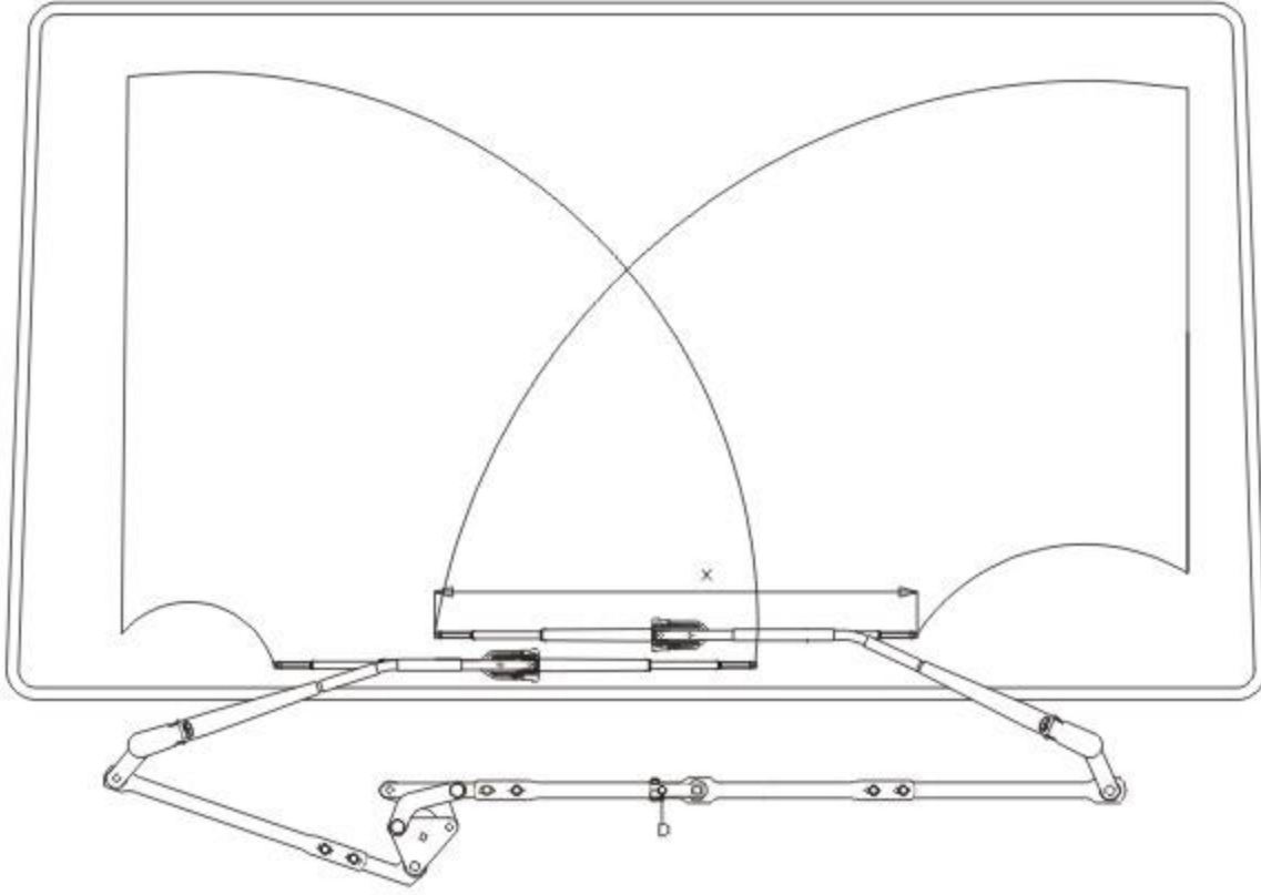
103045 SAĞ KOL KISA
