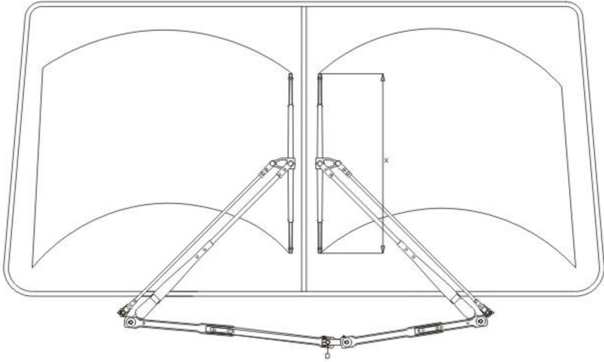
105145 SİLGİ KOL GRUBU
