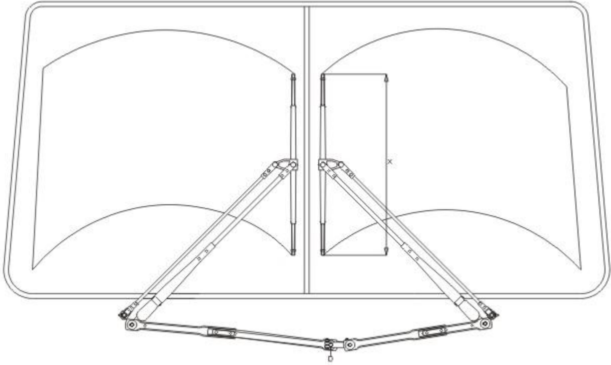
105164 SİLGİ KOL GRUBU
